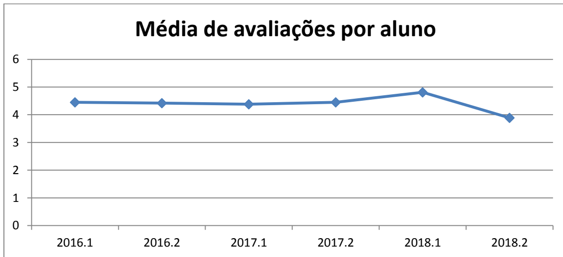
Figura 1: Média de avaliações por aluno de 2016.1 a 2018.2. Fonte: Sig@.
